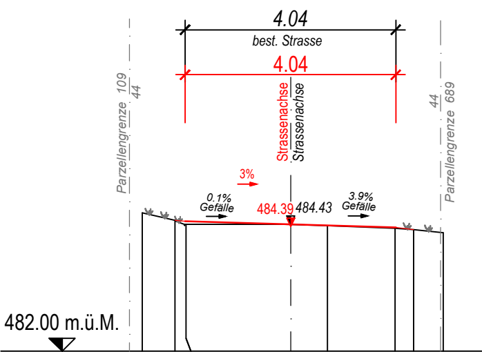
Querprofil 100.00m
