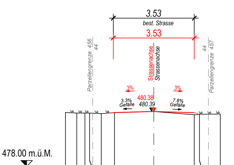
Querprofil 500.00m
