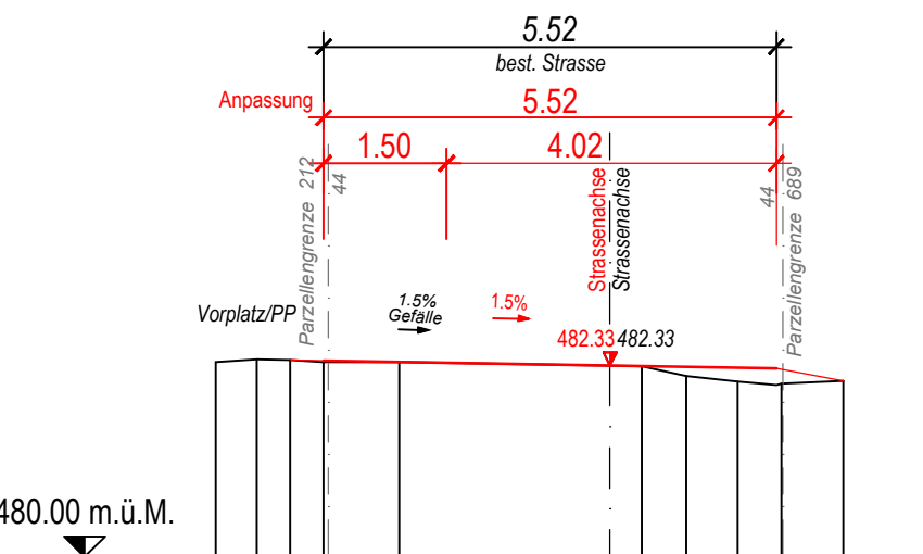
Querprofil 200.00m
