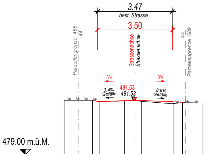
Querprofil 300.00m
