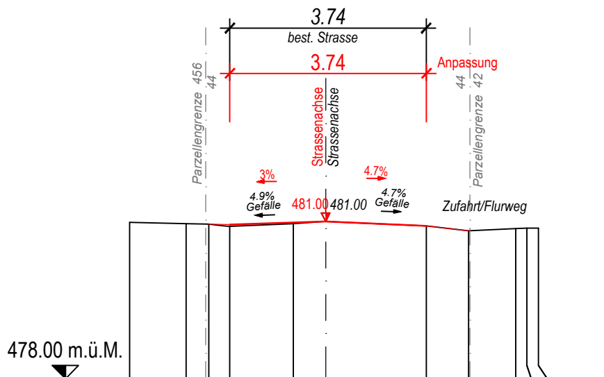
Querprofil 400.00m
